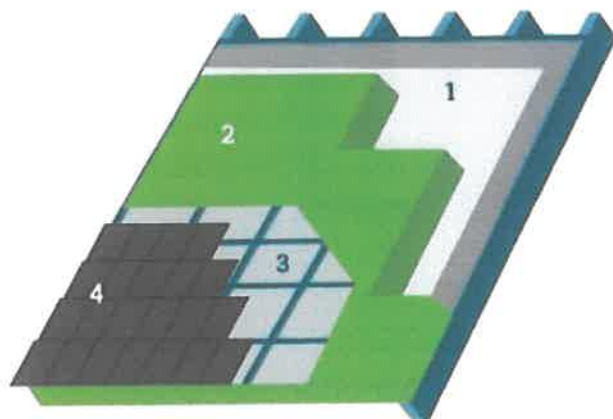
1. Dampscherem | 2. Isolatie | 3. Onderdak | 4. Dakbedekking
